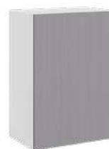
Шкаф навесной (1 дверь глухая) → 1 7 1 ↑ 500|314|720
